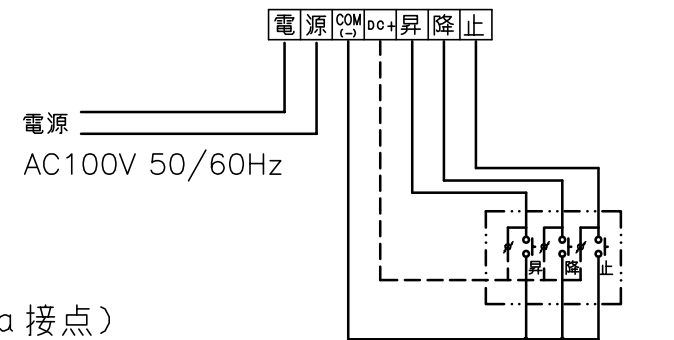
結線図
