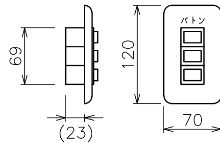
一連壁埋込スイッチ (オールα接点)
