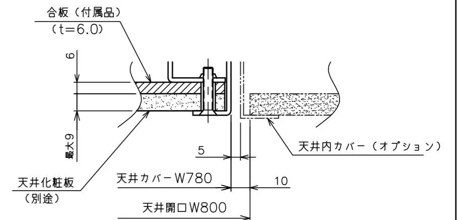
'A'部断面
