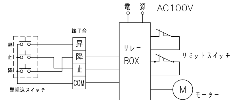
結線図
