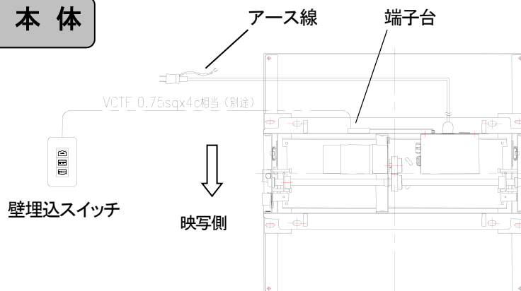
■ 上から見た図 (※イラストはEEP-025M11)
