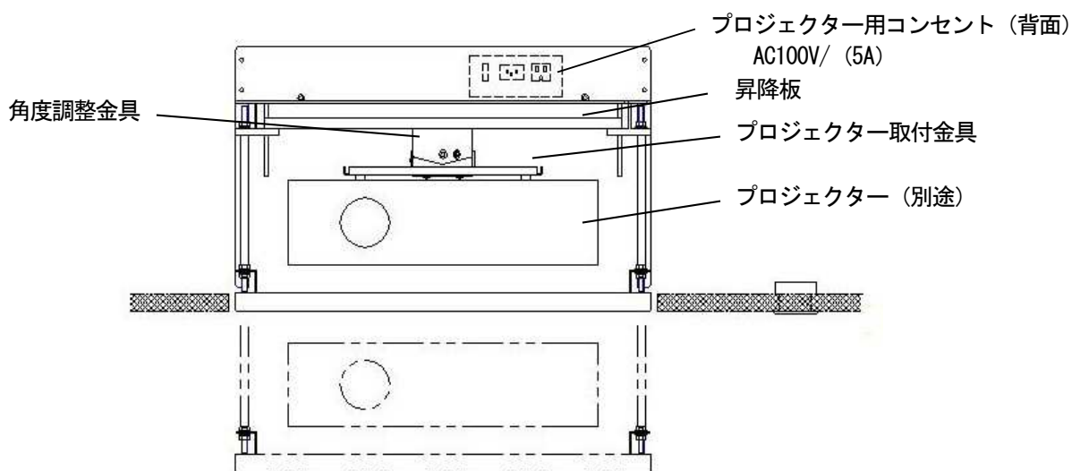
■ 前から見た図 (※イラストはEEP-025M11)
