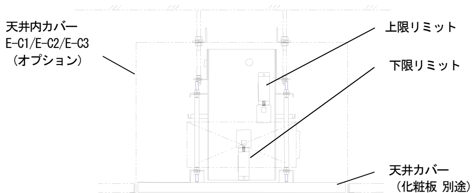
■ 横から見た図 (※イラストはEEP-025M11)
