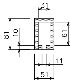
断面図 A-A
