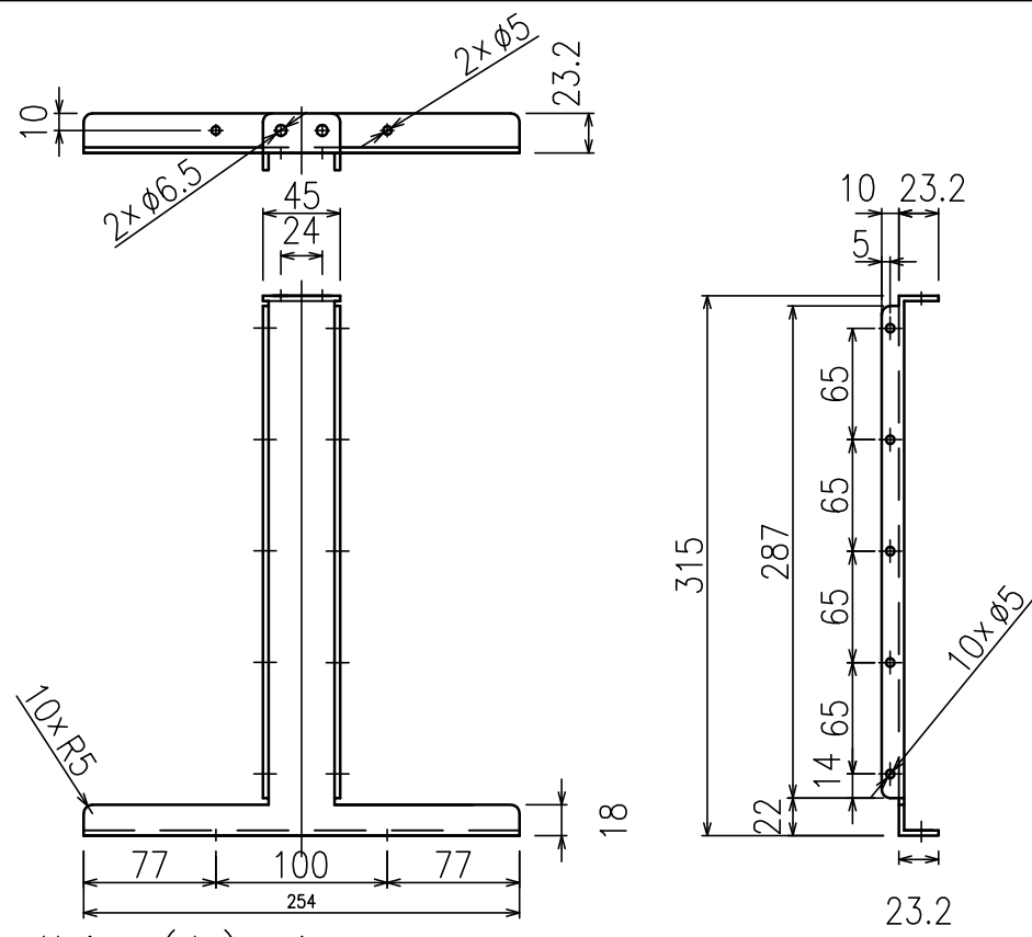
取付金具(大)×1
