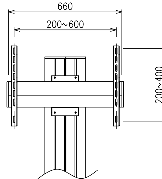
ディスプレイ取付部詳細図
